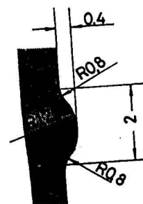
Detalle Y E/ 10:1
