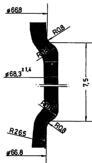
Detalle Z E/ 10:1
